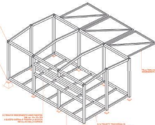
SCHEMA TELAIO
